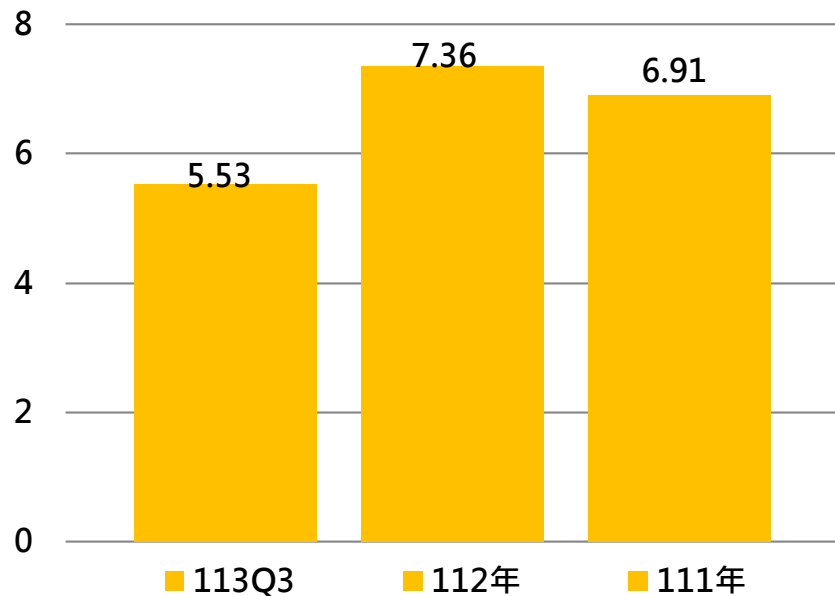
每股盈餘
