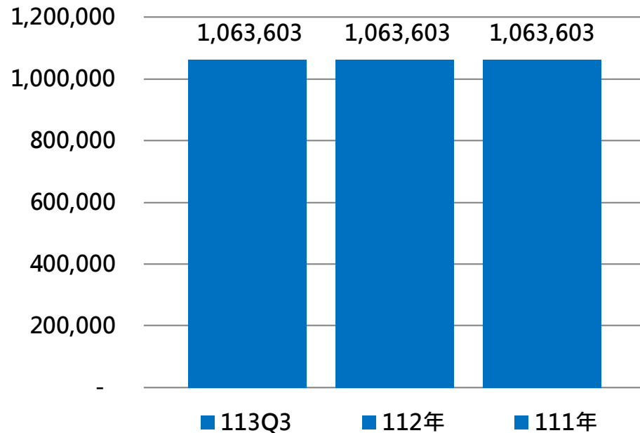
股本
